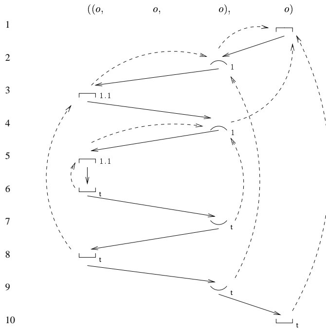
FIG. 12. Trace of F \cdot \text{l-or} .
